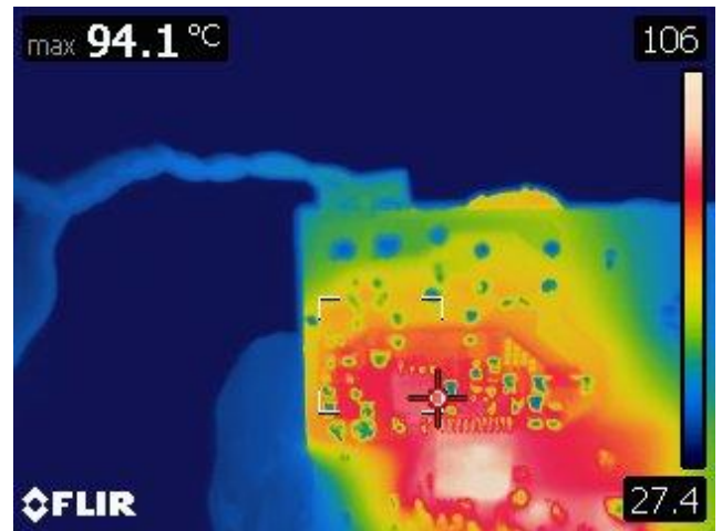
Figure 20 – SR-FET (Q1).
